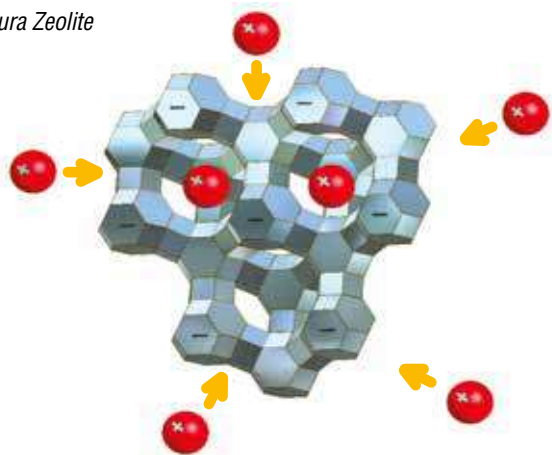
Struttura Zeolite
